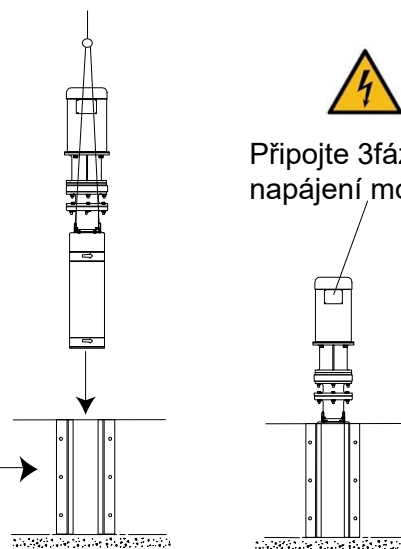
Kanálová montáž
