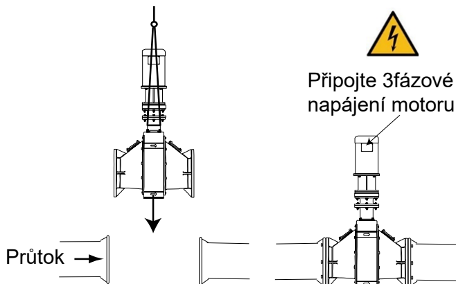
Řadová montáž
